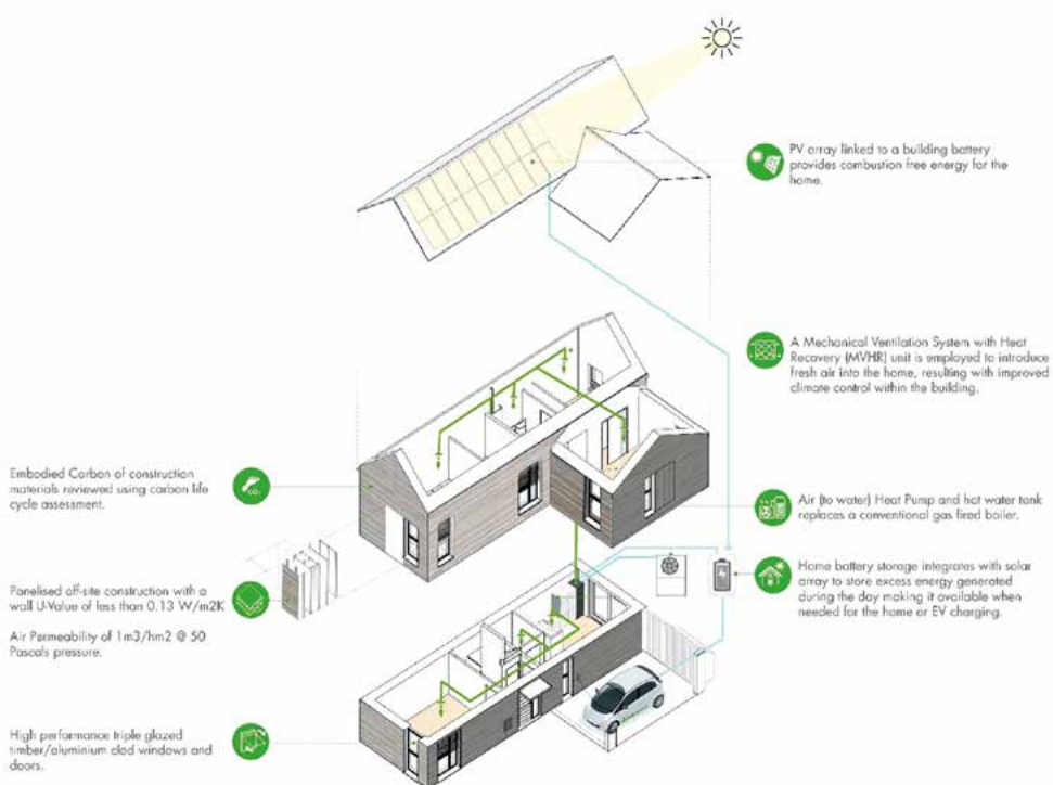
Ffigur 8: Darluniad o'r prif nodweddion dylunio ynni isel
